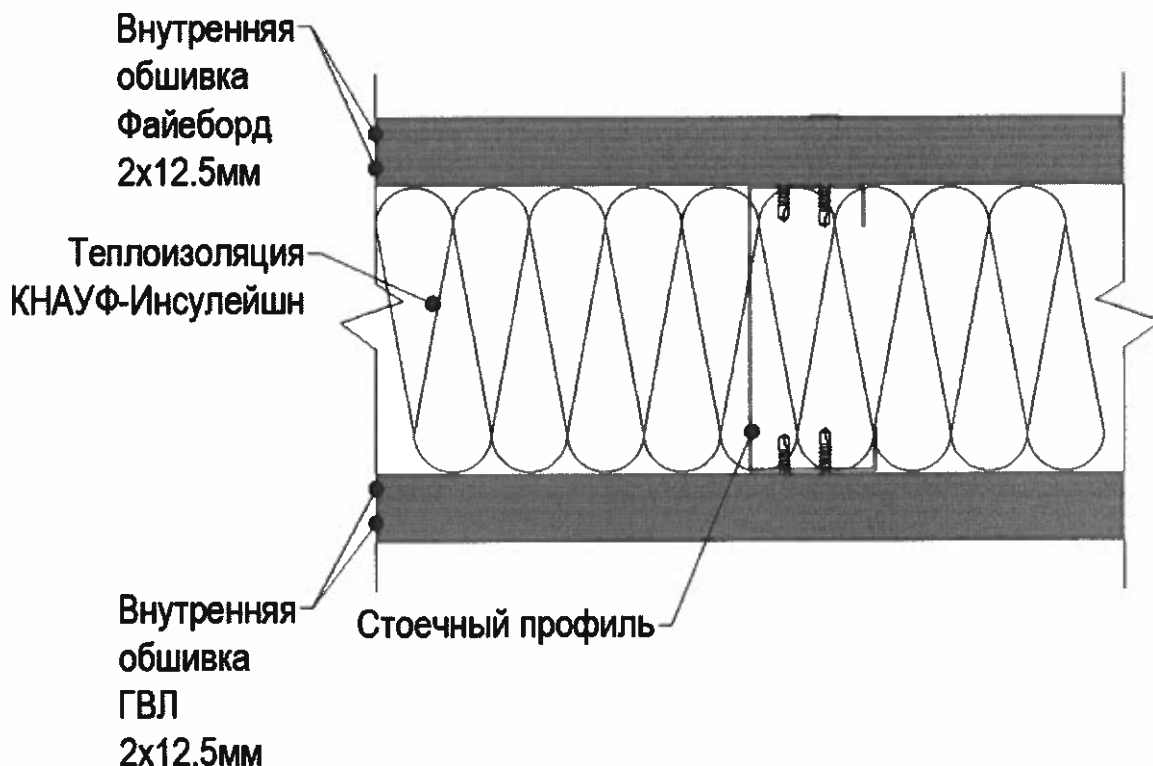
Рис. 8. Конструкция внутренней несущей стеновой панели. Требуемые показатели REI 90, K0(45)
