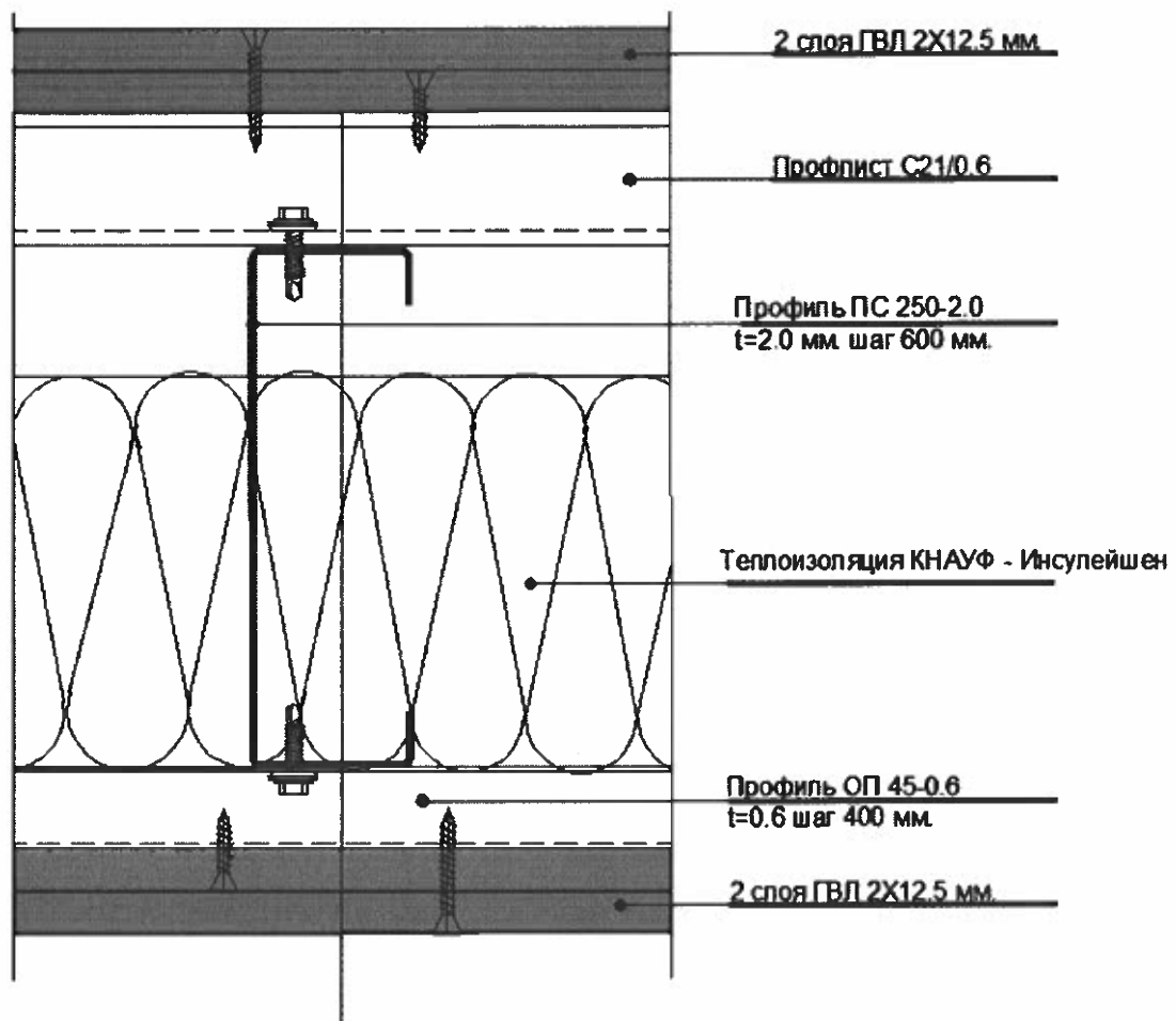
Рис. 10. Конструкция междуэтажного перекрытия. Требуемые показатели REI 45, K0(45)
