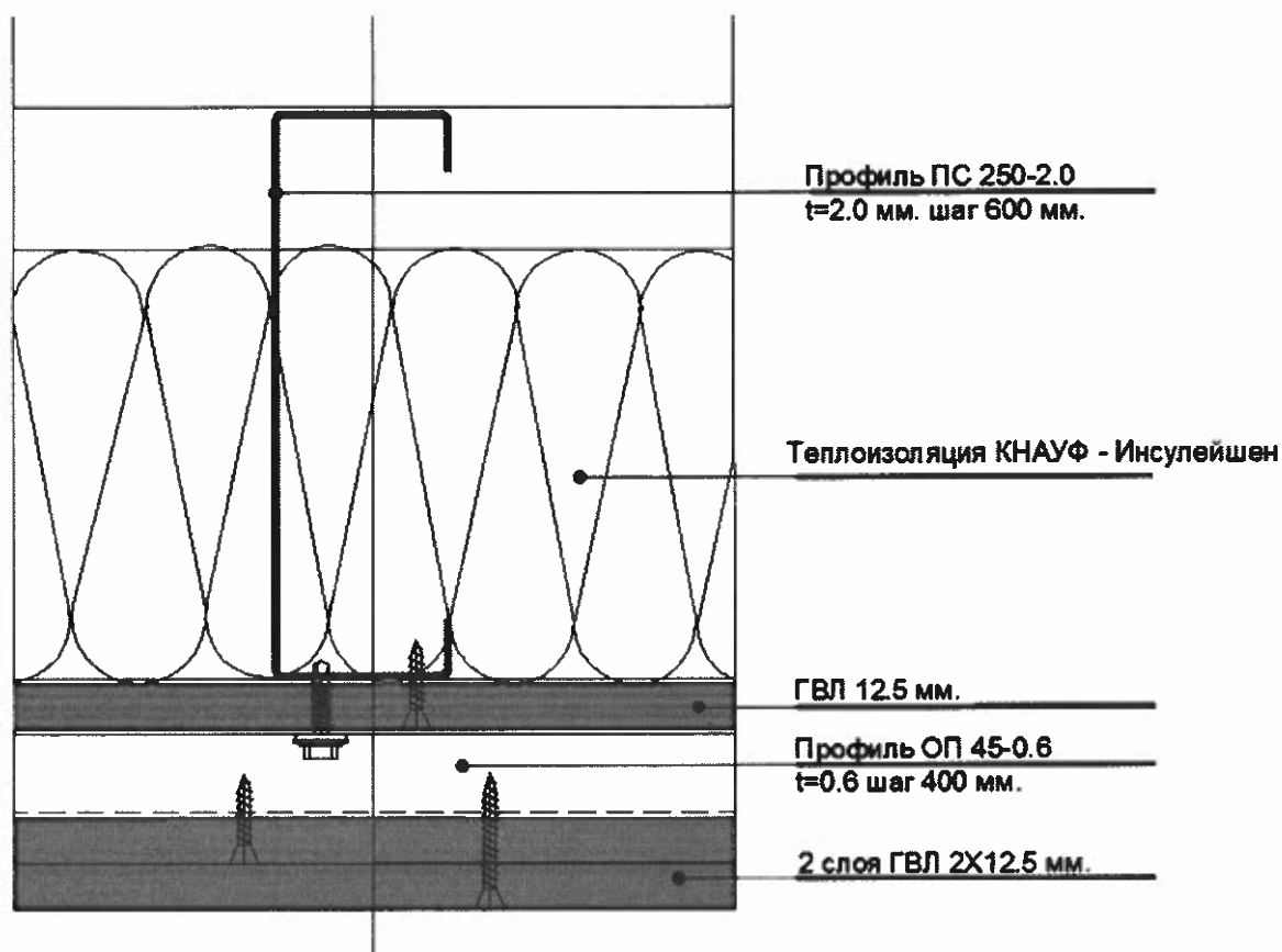
Рис. 10. Конструкция междуэтажного перекрытия. Требуемые показатели REI 90, K0(45)
