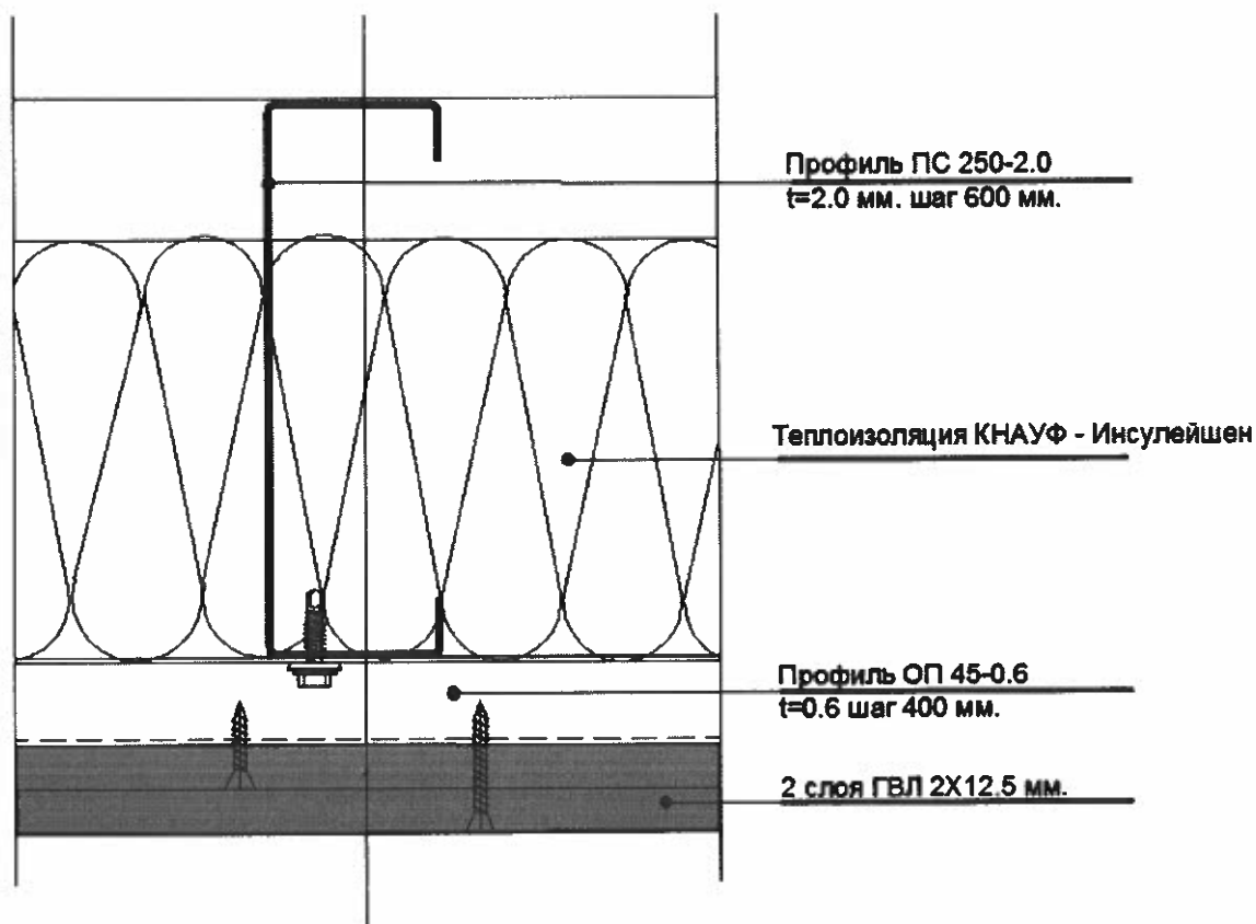
Рис. 11. Конструкция междуэтажного перекрытия. Требуемые показатели REI 45, K0(45)
